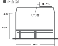
●正面図
